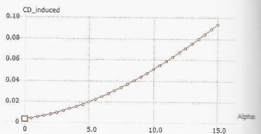
Gambar 14. Variasi AoA terhadap karakteristik aerodinamika pada sayap Cessna 172 R tanpa Winglet
