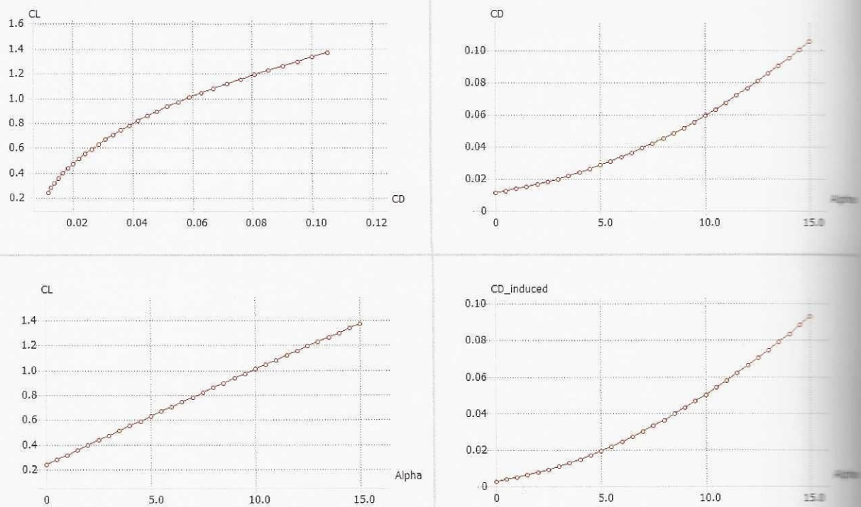
Gambar 17. Variasi AoA terhadap karakteristik aerodinamika pada sayap Cessna 172 R dengan cant angle 90°
